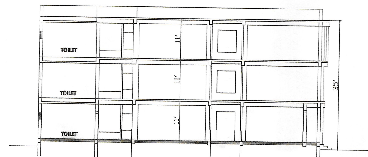
SECTION Y - Y
